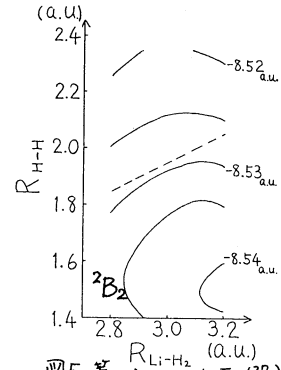
図5. 等エネルギー曲面 ( 2B_2 ) 破線: 2A_1 曲面との交叉線
