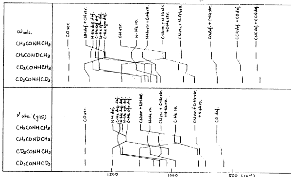
図2 Nメチルアセトアミドの基準振動
