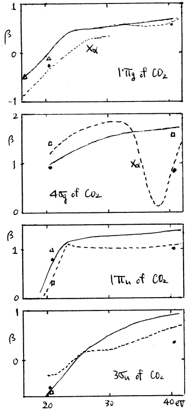
図2 CO 2 の asymmetry parameter (●や△, □は実験値)
