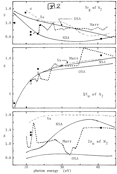
図1. 光イオン化断面積 図2. 異性性パラメータ \beta ○は実測値 (Marr 実測) □は本文参照
