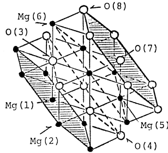
図 2 Mg_{13}O_{13}
