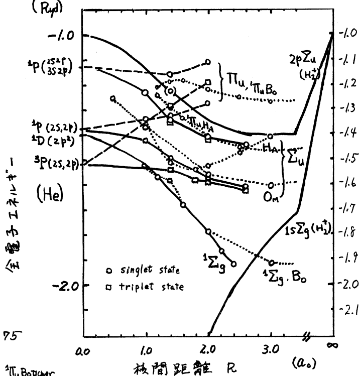
図1. 2電子励起共鳴状態、エネルギー準位
